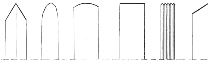
Keilschliff
